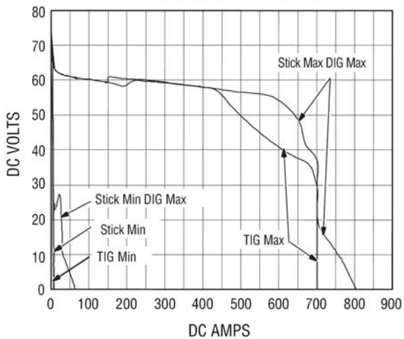
CURVA DE VOLT/ AMP DC
