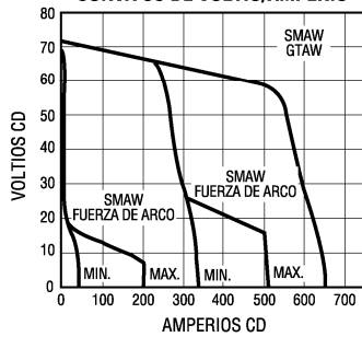
CURVA CC DE VOLTIO/AMPERIO
